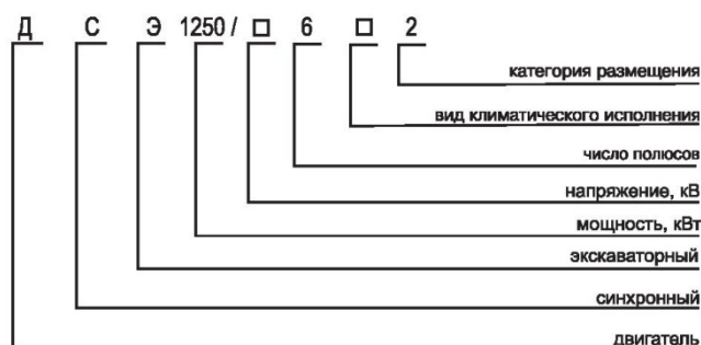
Структура условного обозначения двигателей серии ДСЭ
