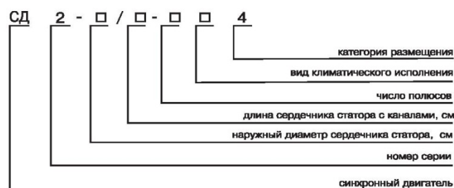
Структура условного обозначения двигателей серии СД-2, 380 В
